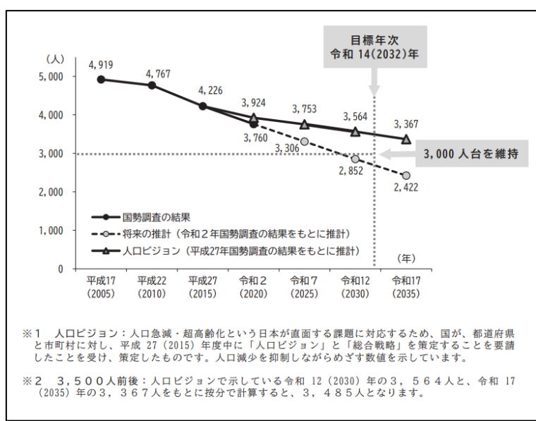
図5 第6次鹿部町総合計画が示す鹿部町の人口推計
