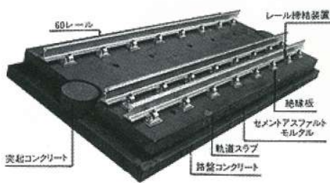
■3線式スラブ軌道
