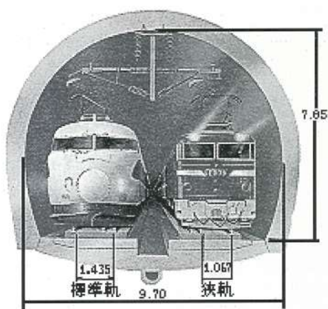
■複線新幹線型トンネル断面
