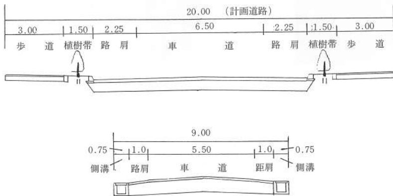
(図1) 国道278号線、鹿部町拡幅計画幅員構成予想図
