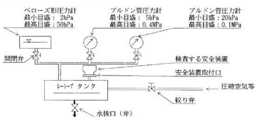
例2 最高試験圧力0.4MPaの試験装置
