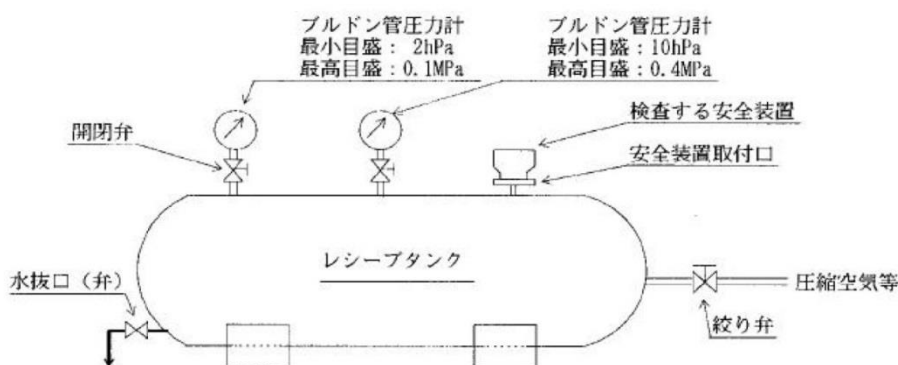
例2 最高試験圧力0.4MPaの試験装置
